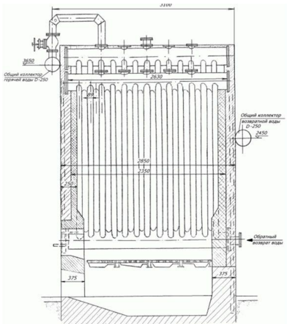
Рис. 2. Котёл ВСТ-5 в продольном разрезе.
