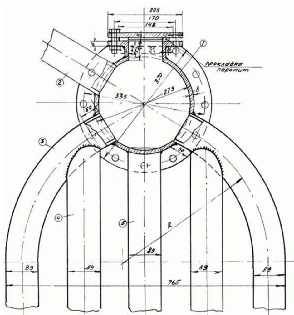
Рис. 3. Трубная часть с коллектором котла ВСТ-5.
