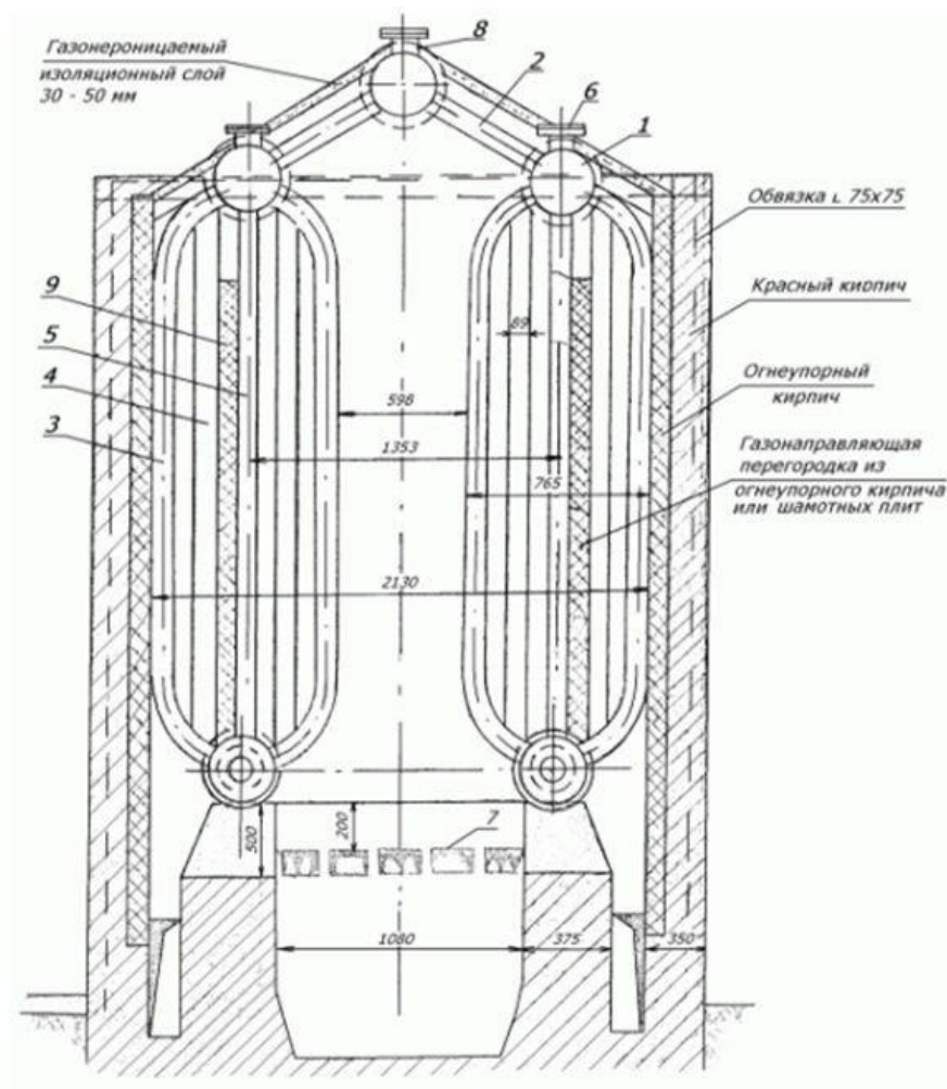
Рис. 1. Котёл ВСТ-5 в поперечном разрезе.
