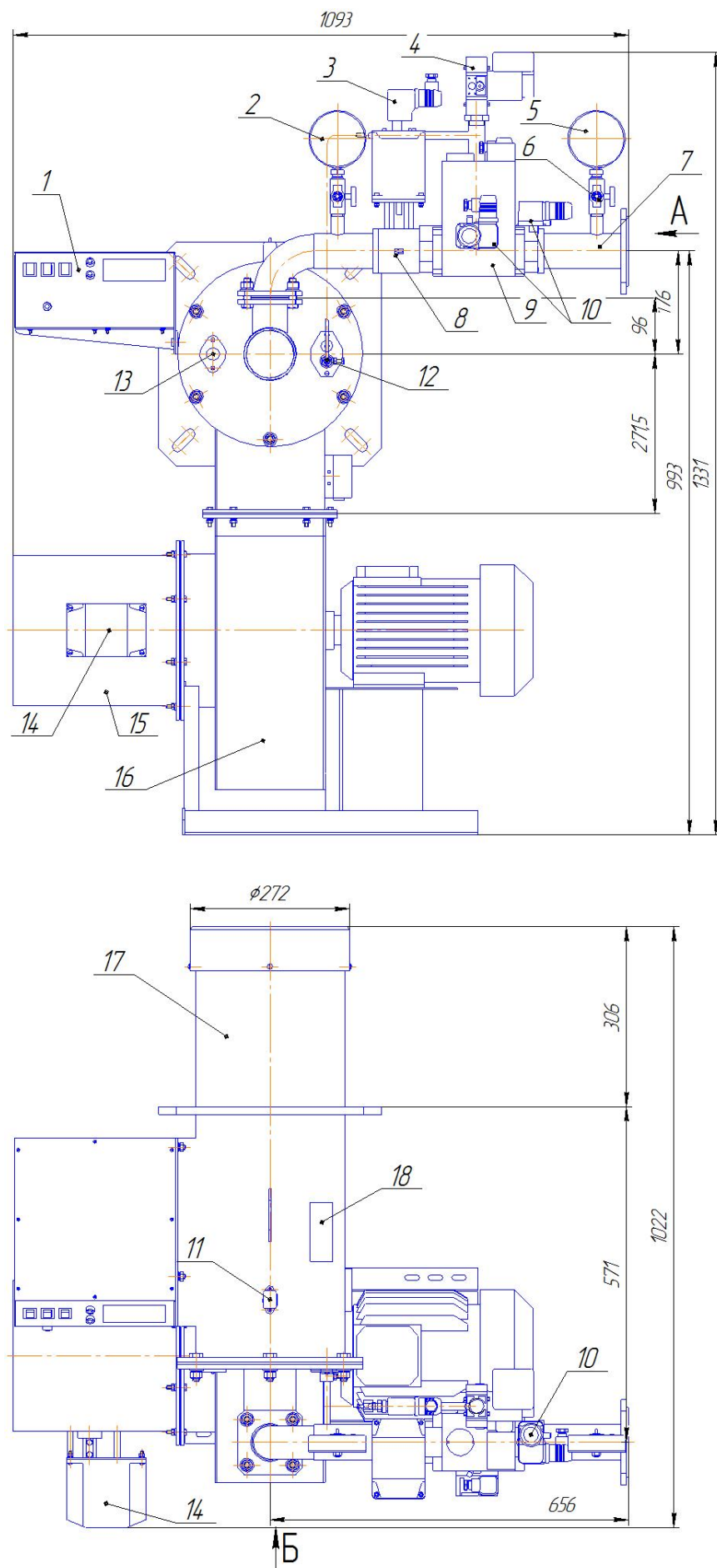
Горелка блочная газовая ГБ-2,4 ГБд-2,4.00.00.000
