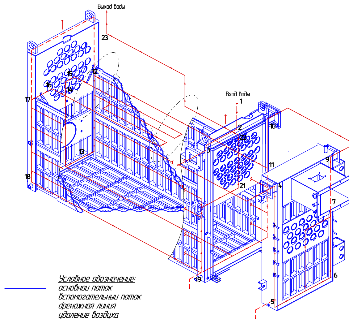
РИС. 3 СХЕМА ГИДРАВЛИЧЕСКАЯ КОТЛА КСВа-0,5
