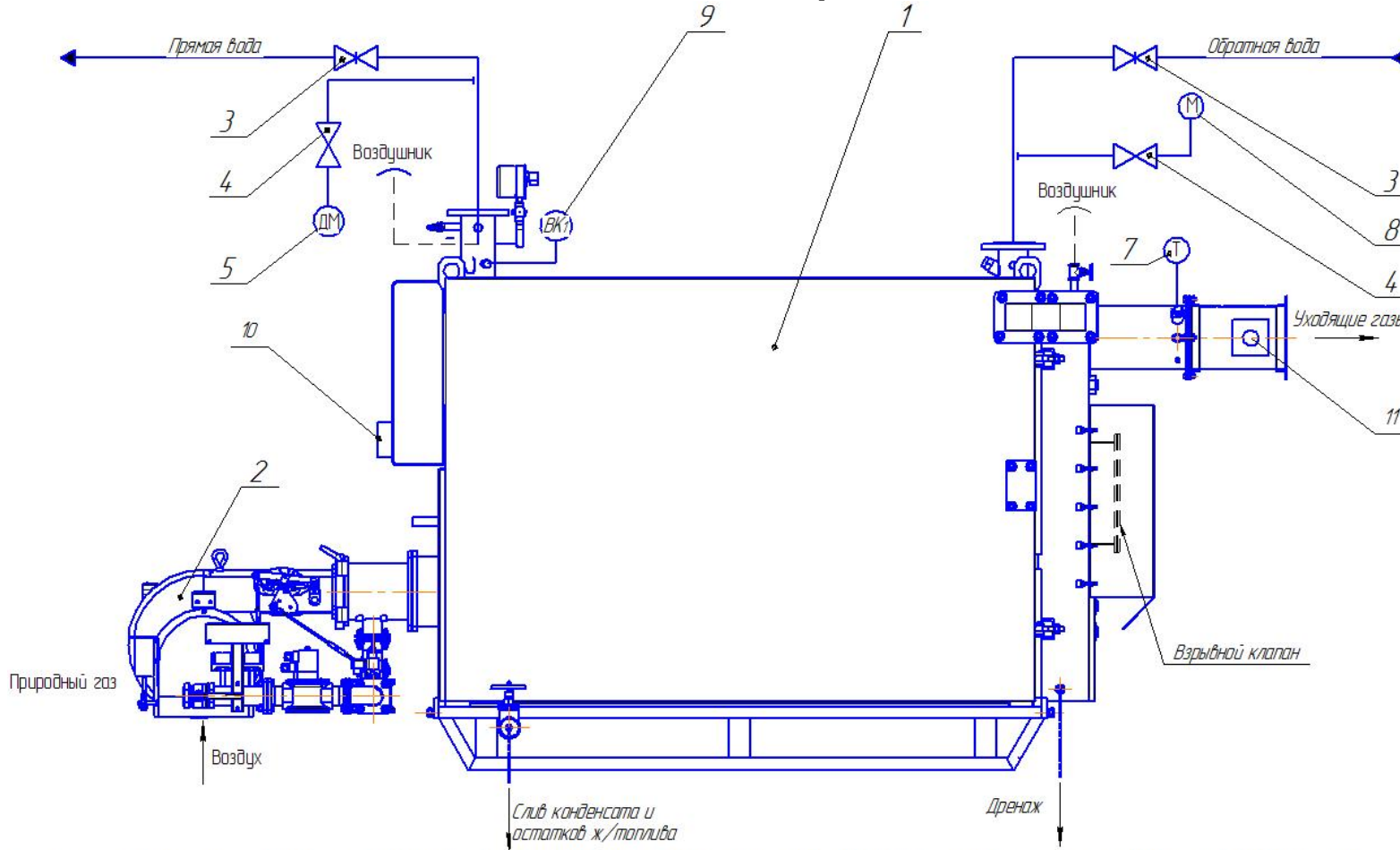
РИС. 1 СХЕМА ФУНКЦИОНАЛЬНАЯ КОТЛА КСВа-0,63
