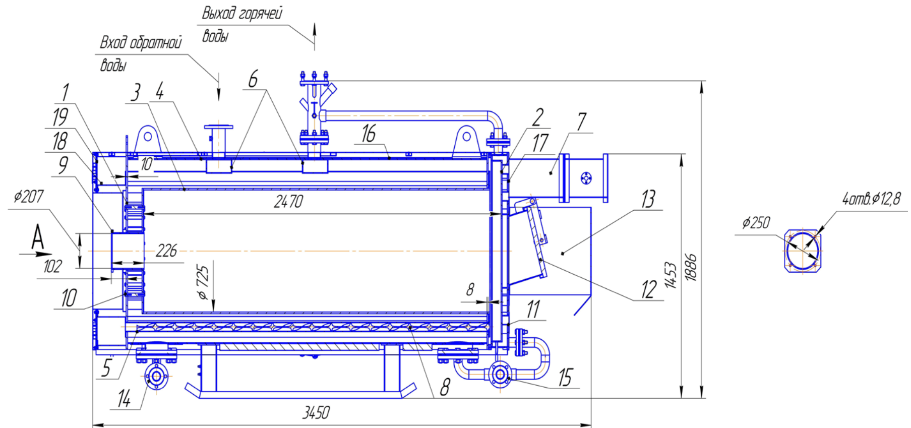
РИС.2. КОТЁЛ КСВа-1,0 В РАЗРЕЗЕ.
