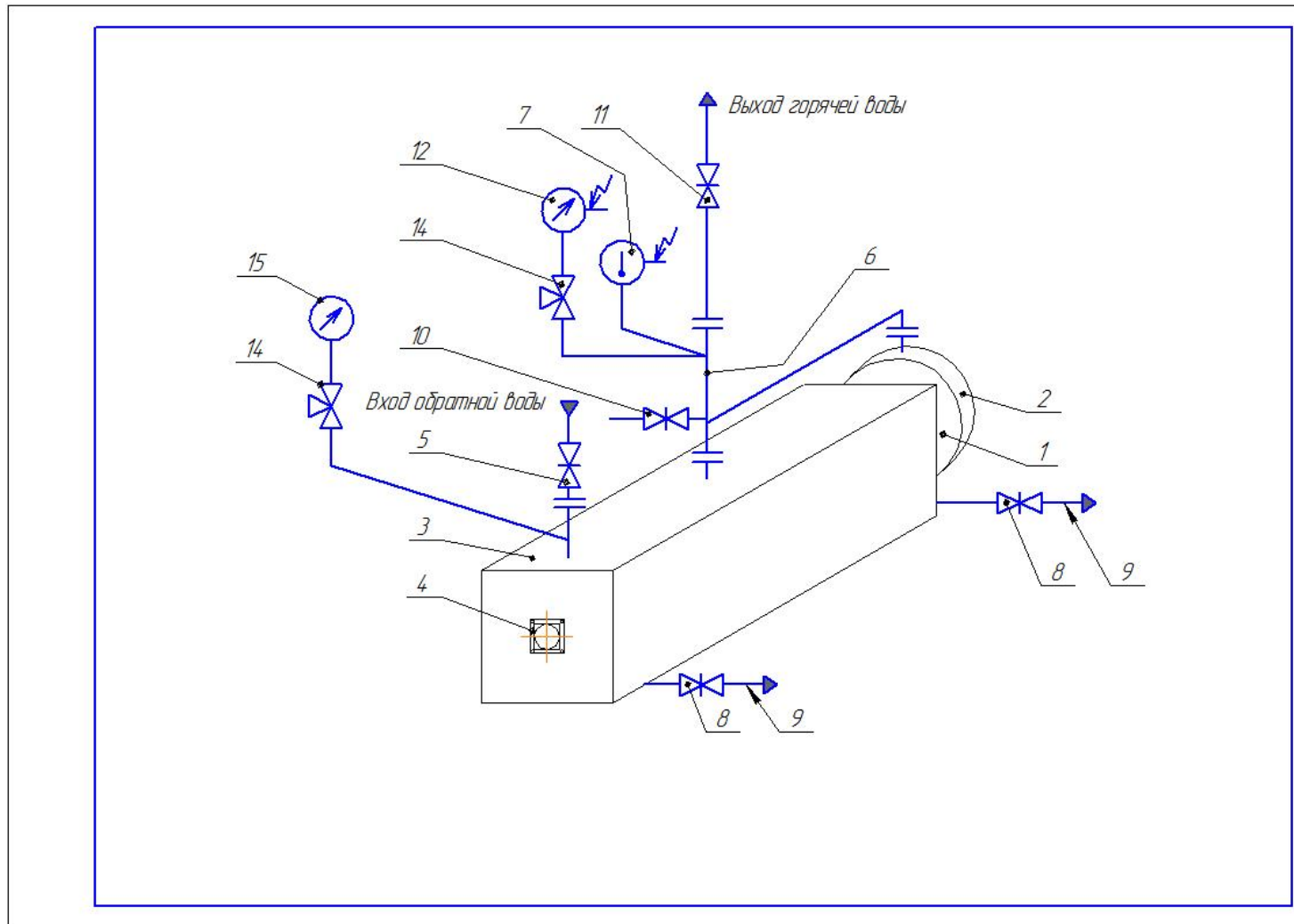
Рис.1 СХЕМА ВОДЯНОГО ТРАКТА КОТЛА КСВа-1,0
