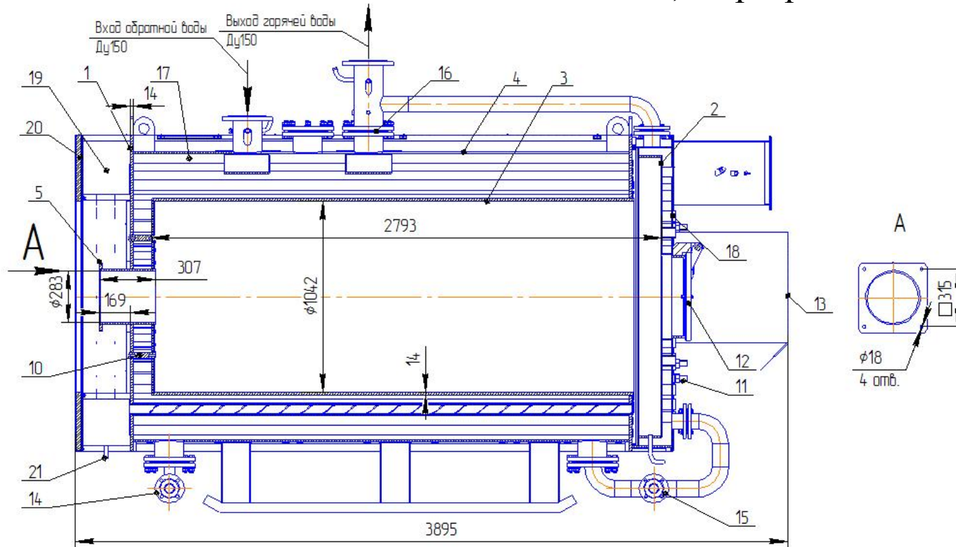
Рис.2. Котёл КСВа – 2,5 в разрезе
